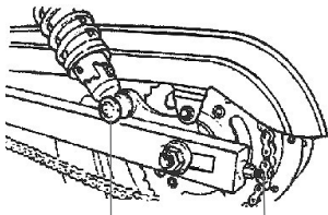
مهره ثابت‌کننده توپی
